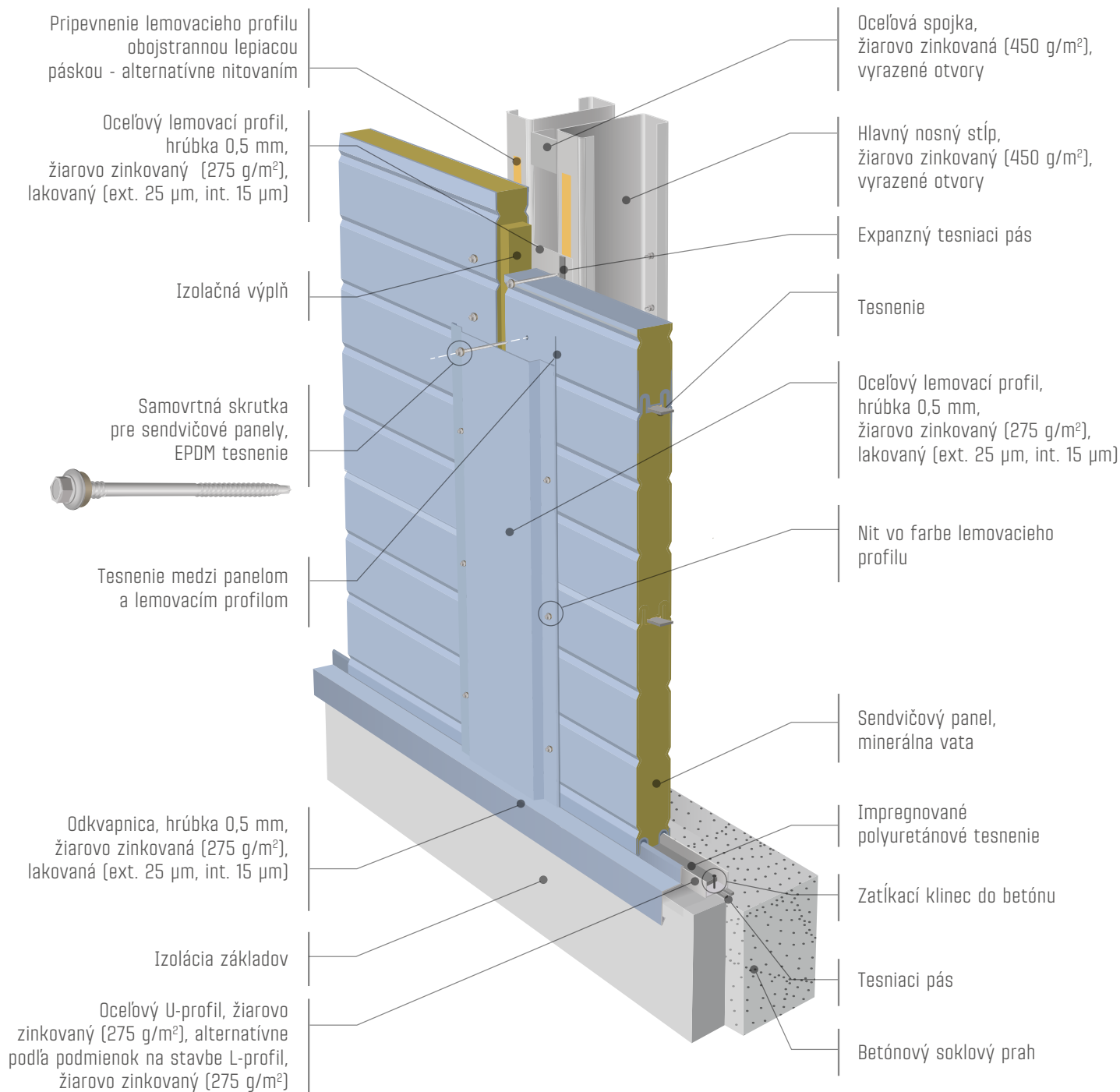
TABUĽKA HODNÔT PRE PANELY - VÝPLŇ Z MINERÁLNEJ VLNY
